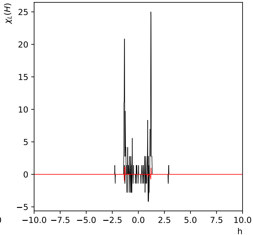
\chi_L(H) réseau de taille L=6 à T=1.5
