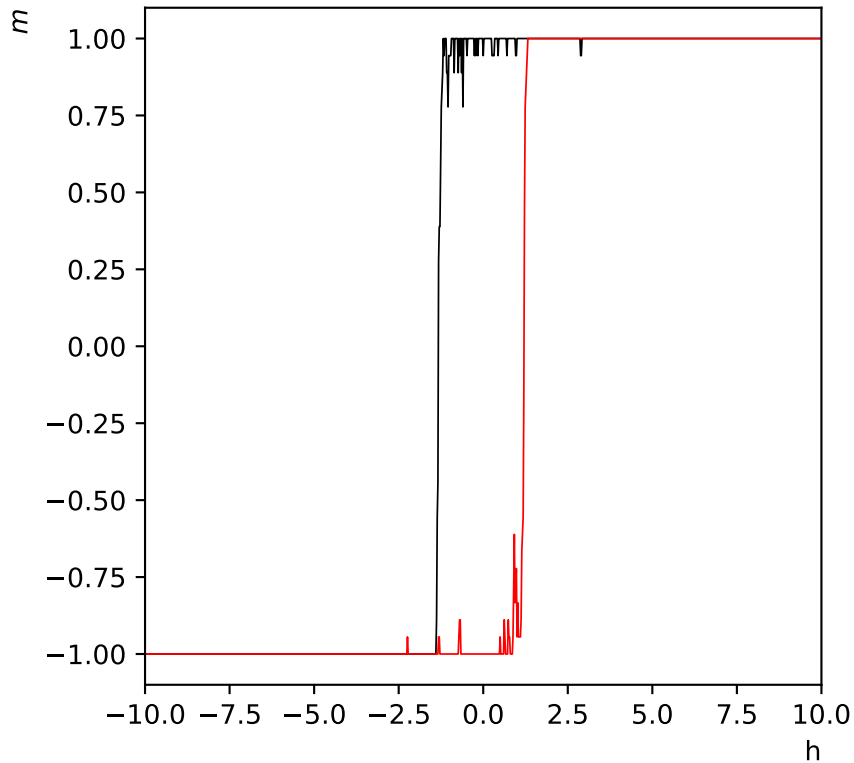
Hystérésis de l'aimantation réseau de taille L=6 - h=10 à T=1.5
